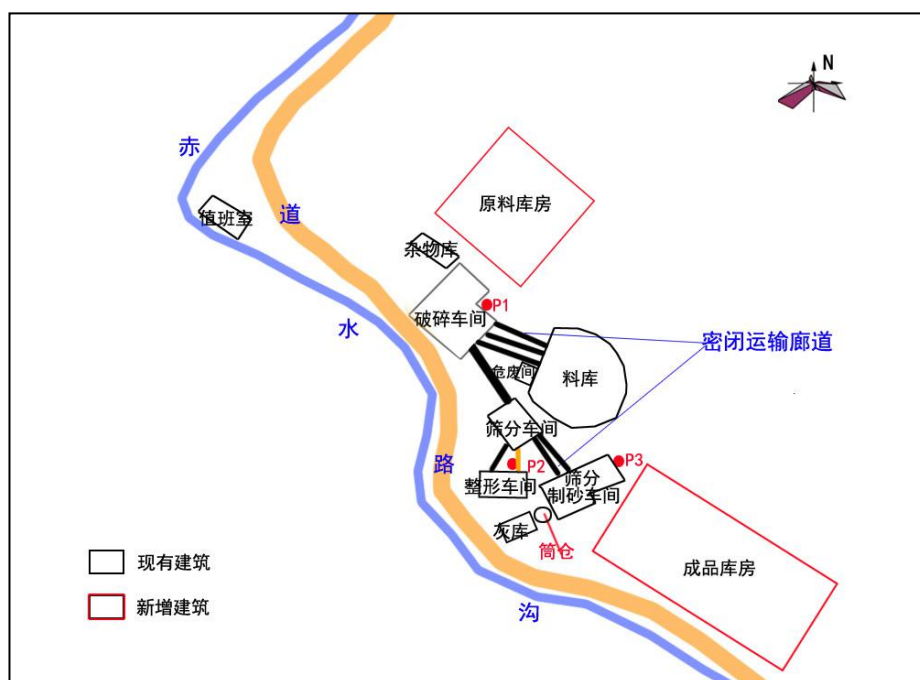
图 2-7 加工区平面布置示意图
