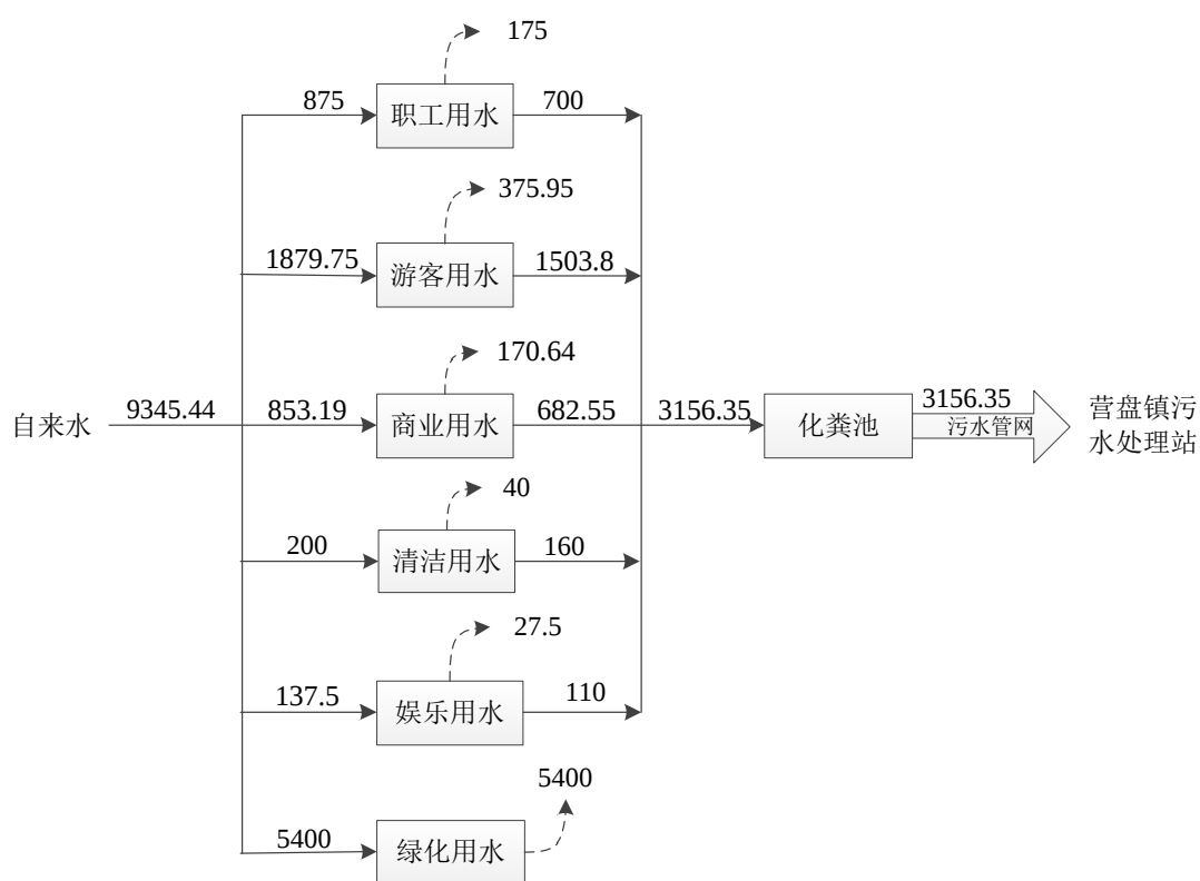
图 2-1 项目水量平衡图 m³/a
