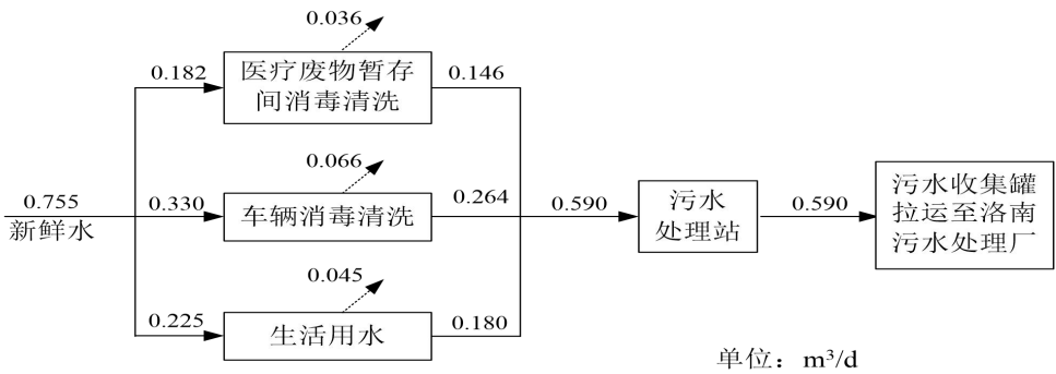
图 2-2 水平衡图
