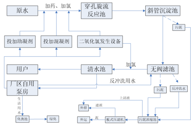
图 2-5 一期净水厂运营期工艺及产污环节图
