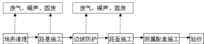
图 2-4 道路施工流程及产污环节
