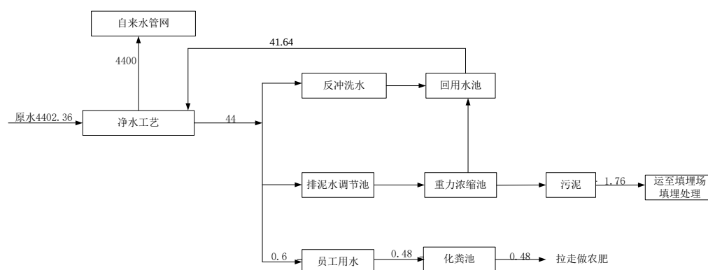
图4-1 项目扩建后全厂水平衡图 单位：m³/d
