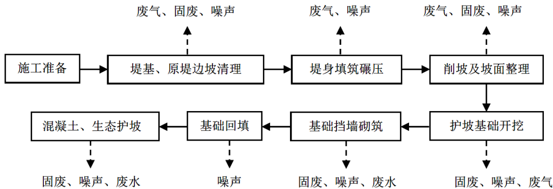
图 2-5 堤防工程施工工艺流程及产污环节图
