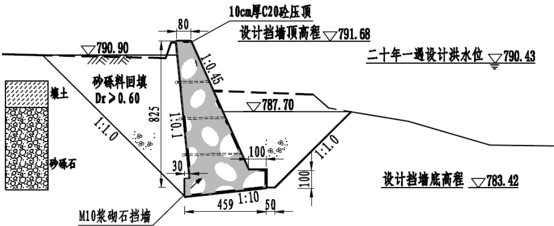
图 2-1 典型设计图
