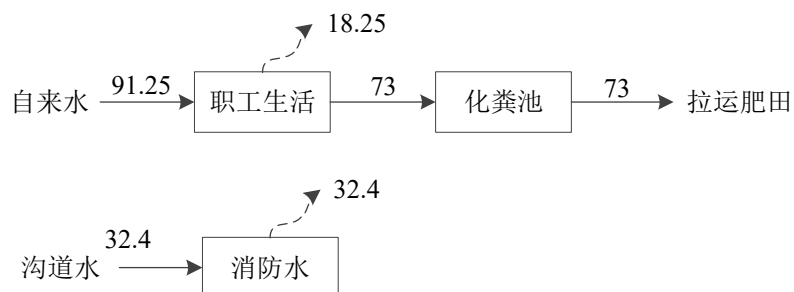
图 2-1 项目水量平衡图 m 3 /a
