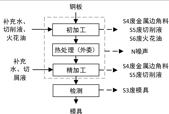
图3 生产工艺流程及产污节点（模具）
