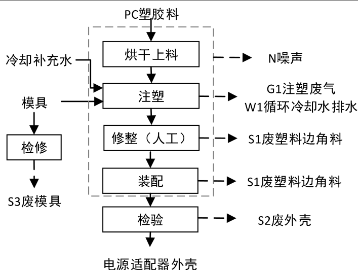
图2 生产工艺流程及产污节点（电源适配器外壳）
