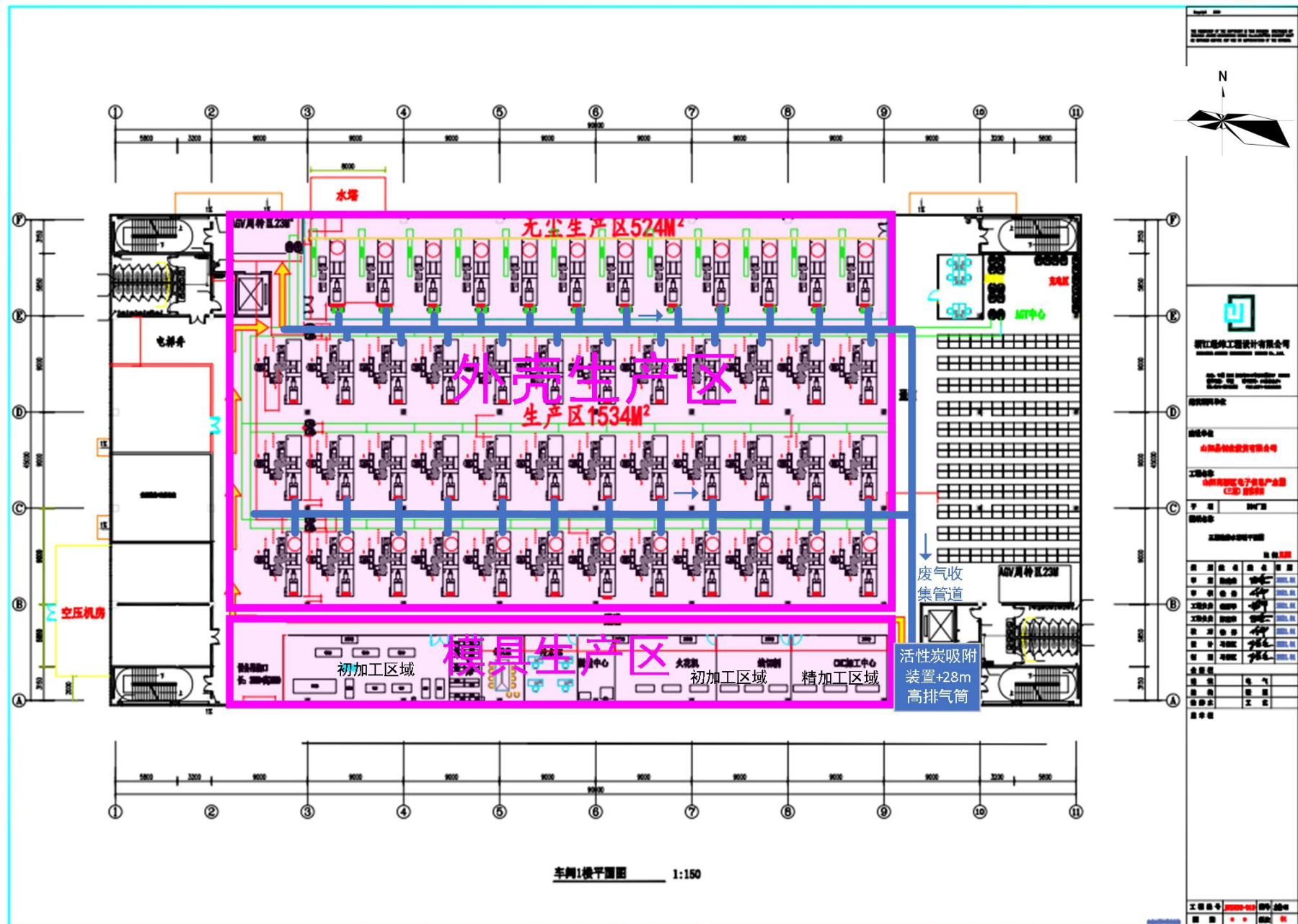
附图 3-1 项目厂区平面布置图 (1F)
