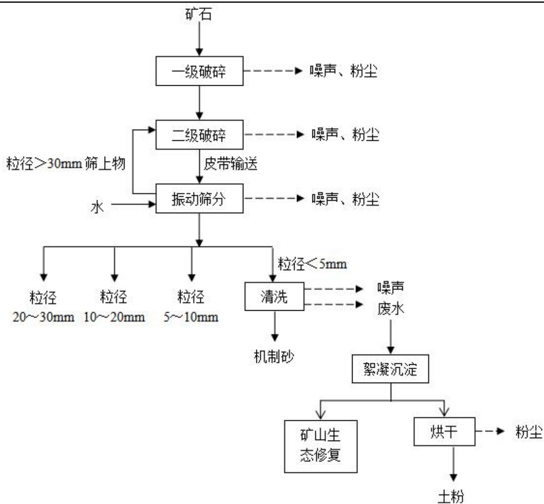
图 2-3 破碎加工工艺流程及产污环节图
